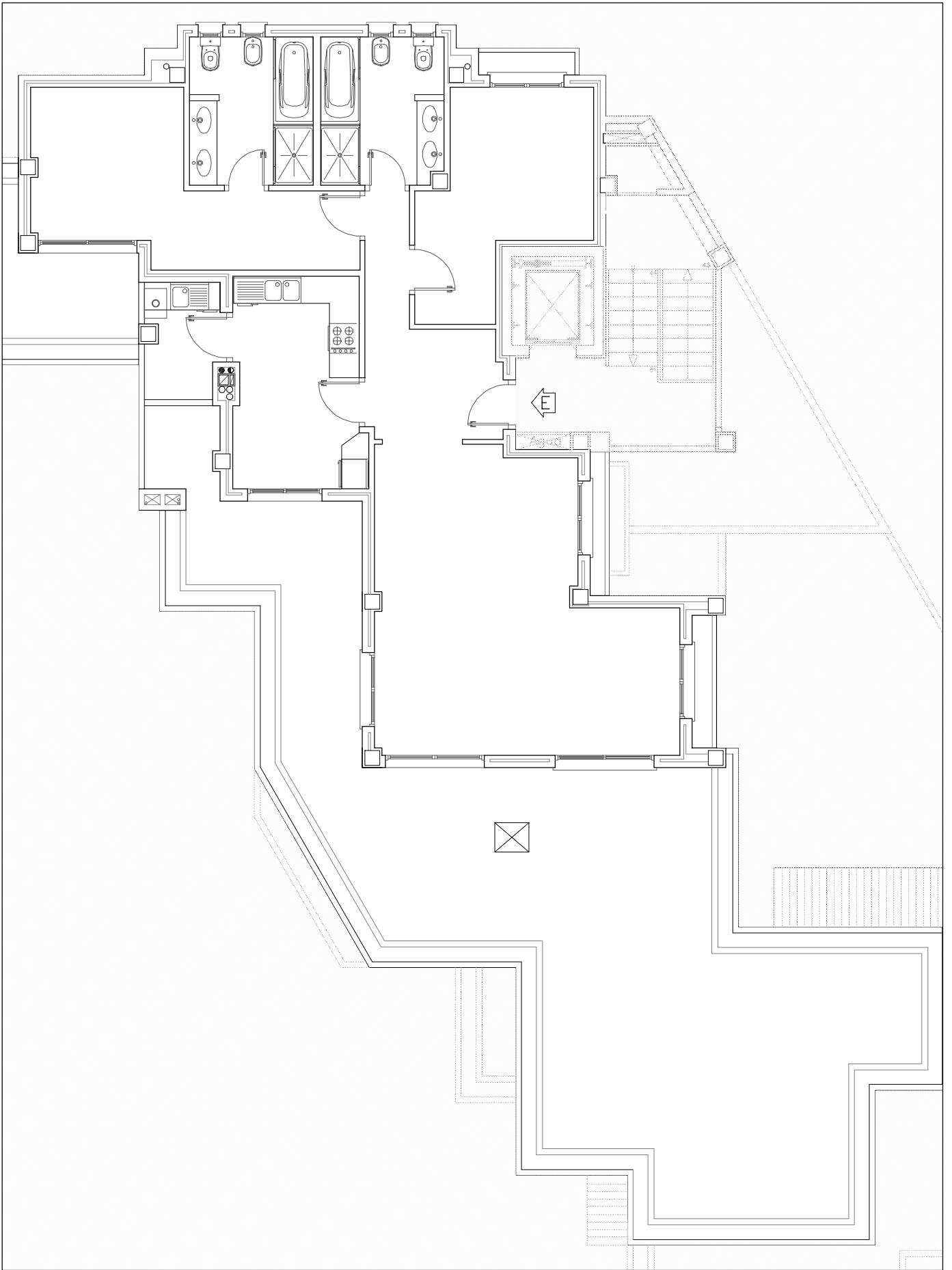
BLOQUE 11 planta ático - vivienda E
